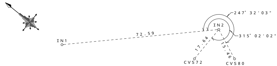
引照点図 S = 1 : 1000
